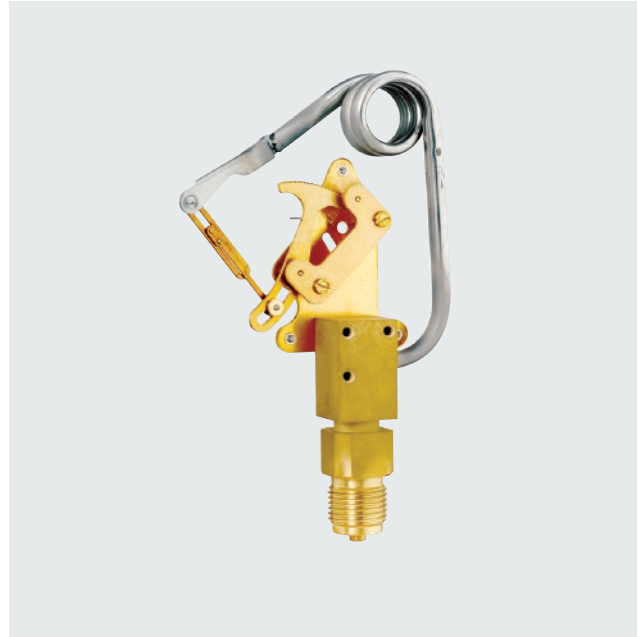
Rohrfeder-Messsystem in Schraubenform
